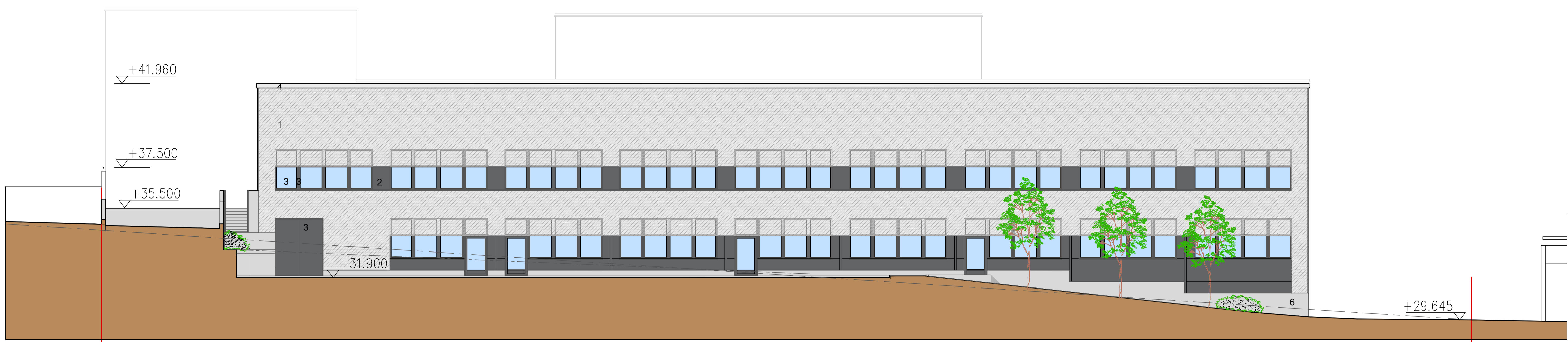
TALO 1, JULKISIVU LOUNAASEEN, HANKASUONTIELLE 1:100
